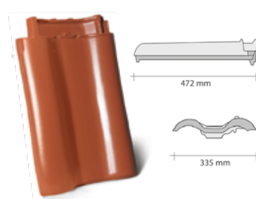
taška s dvojtou návalkou - krycí délka cca: 36,5–40,3 cm - krycí šířka cca: 33,5 cm - hmotnost 1 ks cca: 4,7 kg - používá se jako estetické zakončení levého okraje plochy střechy, namísto základních tašek u kterých by byl vidět zámek. Např. v místě kde střešní plocha navazuje na vyšší stěnu štitu vedlejšího domu.
