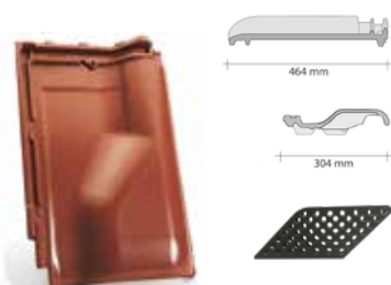
větrací taška
