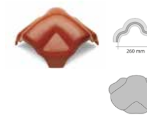
rozbočovací hřebenáč univerzální Y, dostupný je i ve tvaru X nebo T - hmotnost 1 ks cca: 4,8 kg
