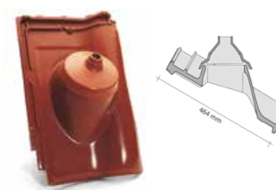
anténní komplet: prostupová
