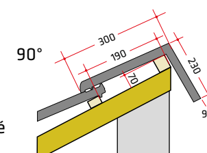
Pultové tašky
